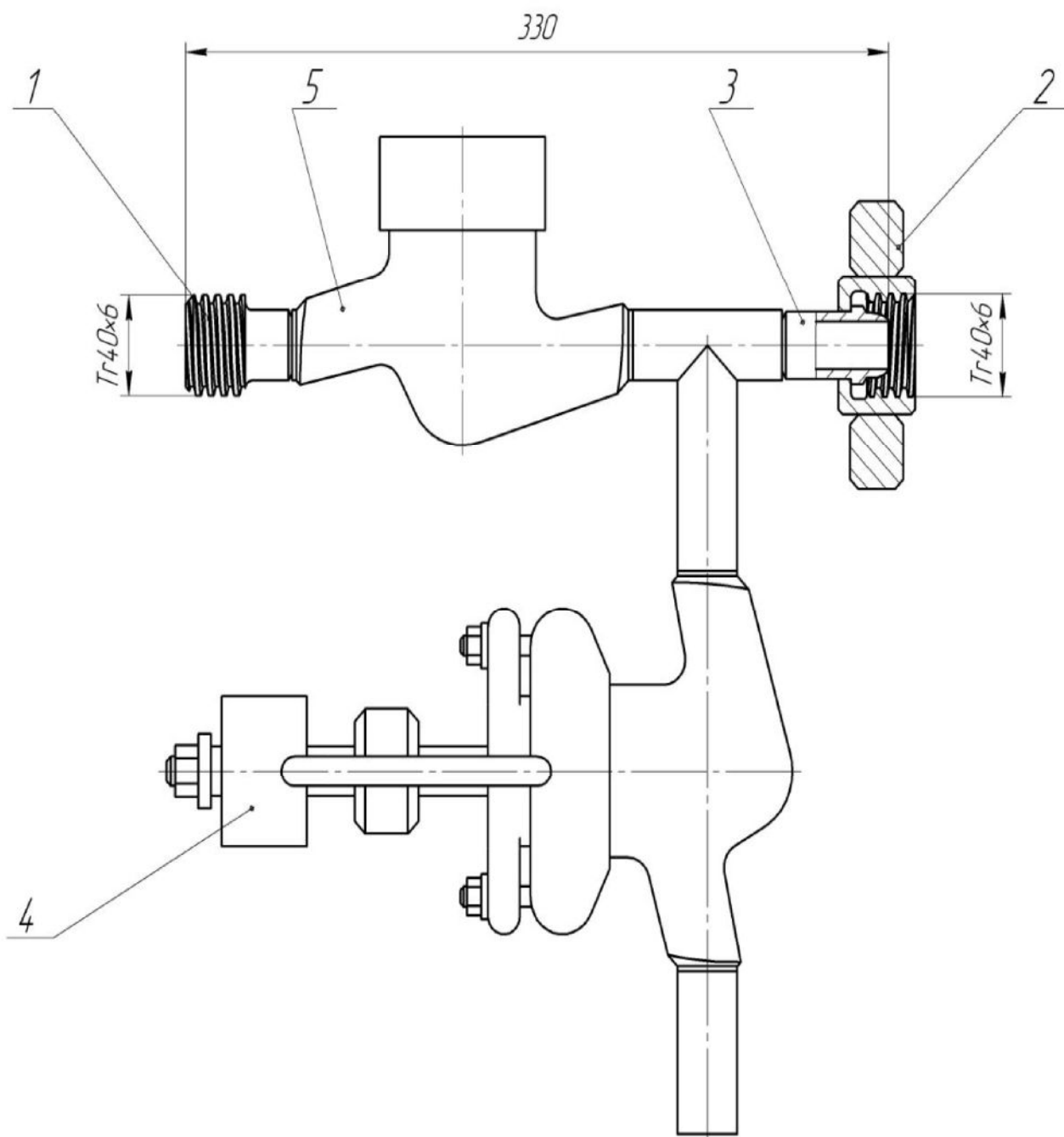
Рисунок 8 – Вентиль запорный
