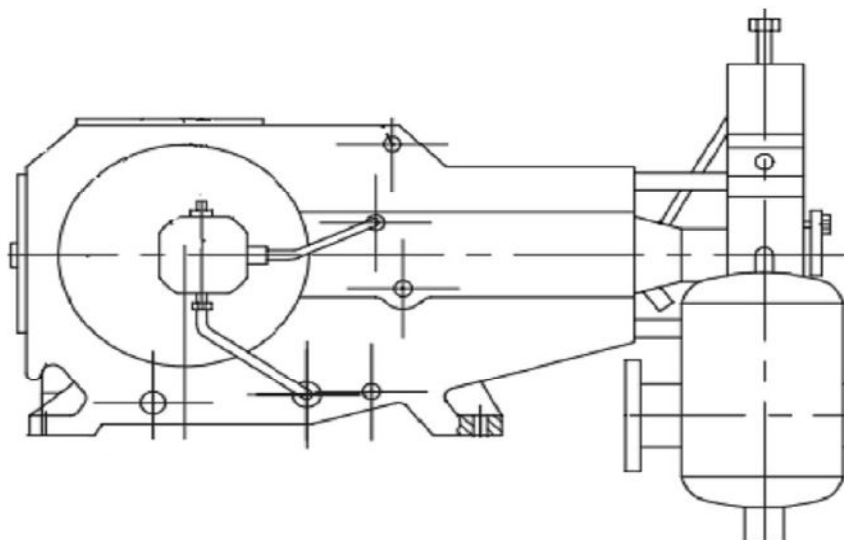
Рисунок 13 - Насос 1.3ПТ-50Д2
