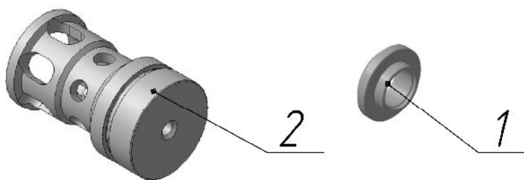
Рисунок 15- Клапан нагнетательный Н500.01.03.000
