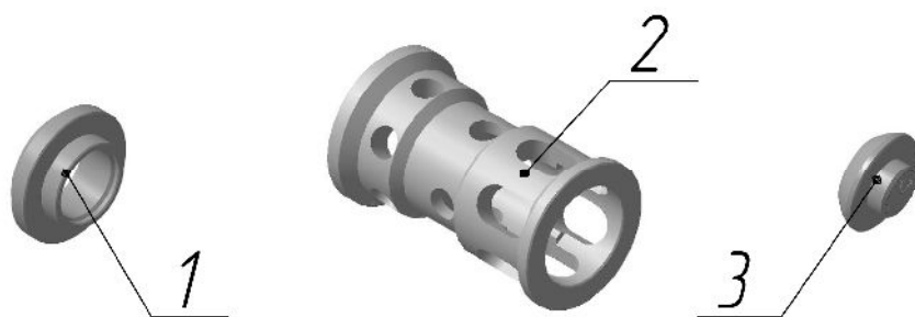
Рисунок 14- Клапан всасывающий Н500.01.03.000
