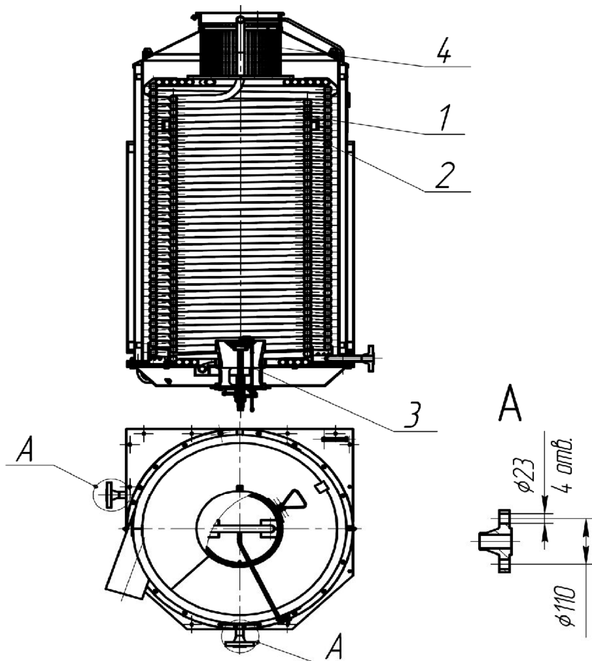
Рисунок 2 -Устройство нагревательное
