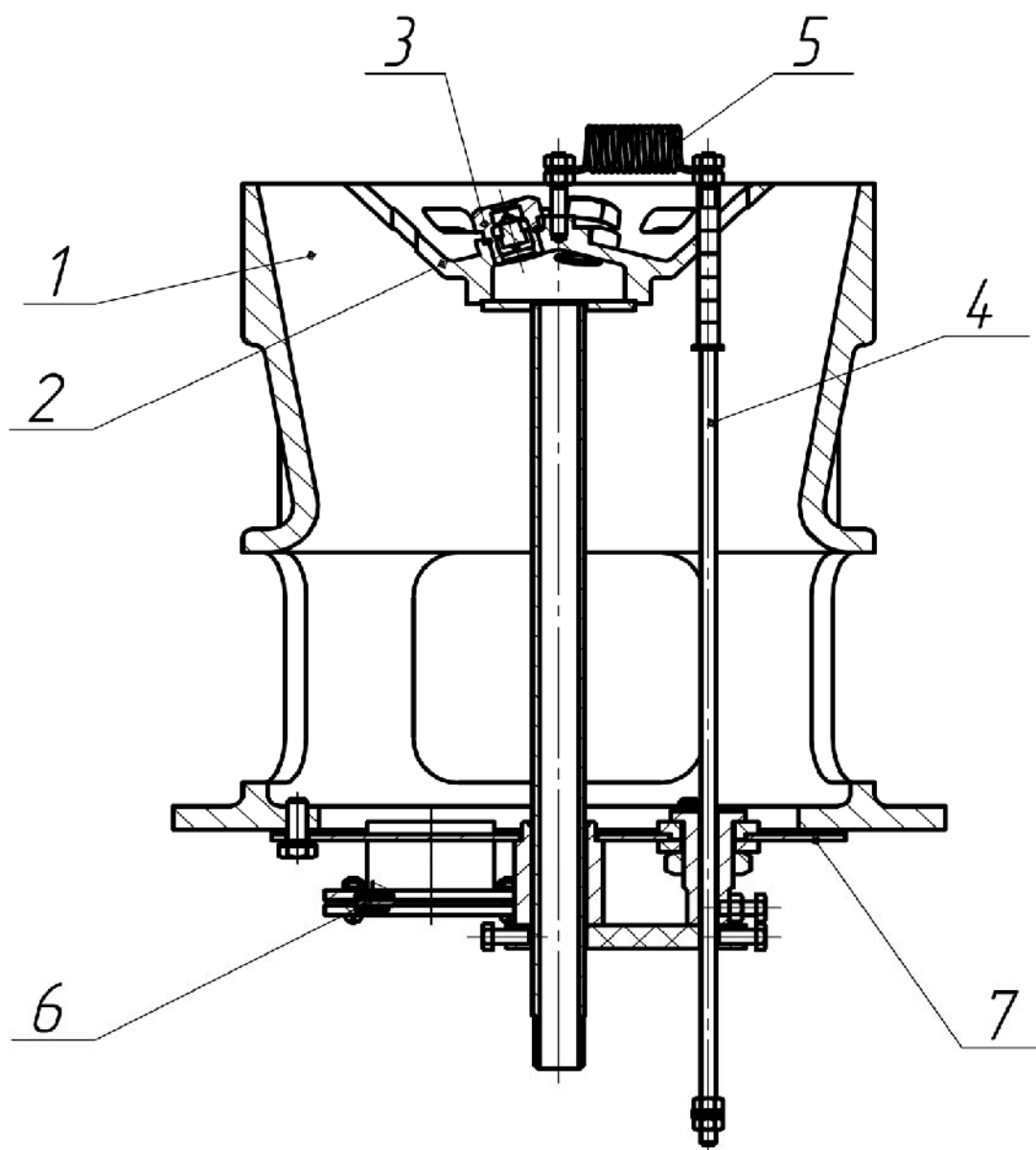
Рисунок 3 -Устройство горелочное трехфорсуночное
