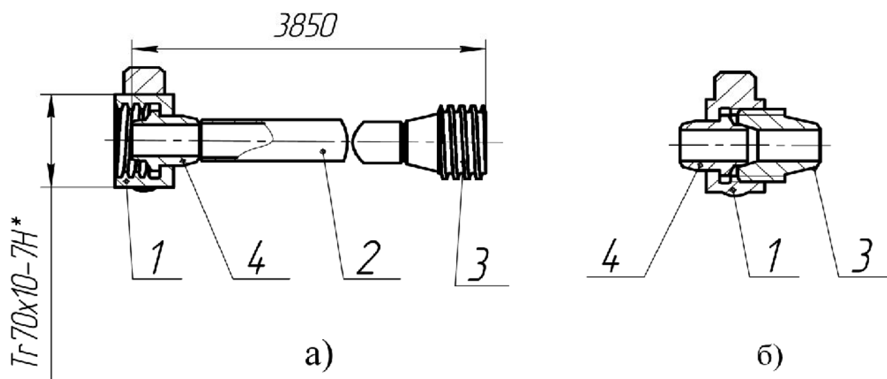
Рисунок 21: а) Труба магистральная Л65.13.01.000 б) БРС АДПМ
